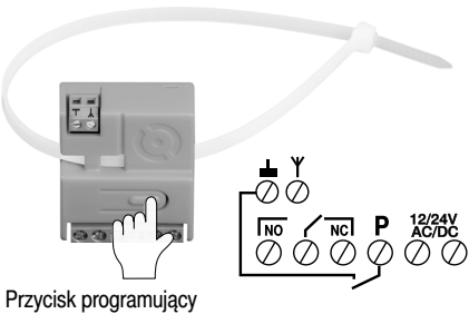
Przycisk programujący
