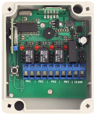
KONTROLER
